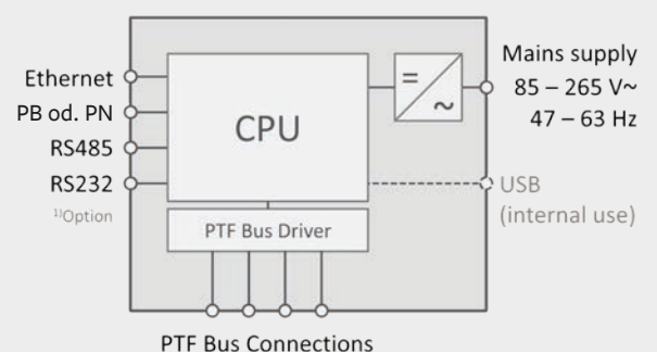
Schéma fonctionnel PTF-SUB3
